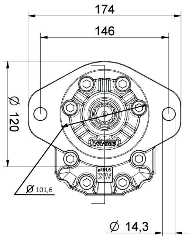
XV3 Ø101,6 SAE B (PRF) (300.0136.AKP)
