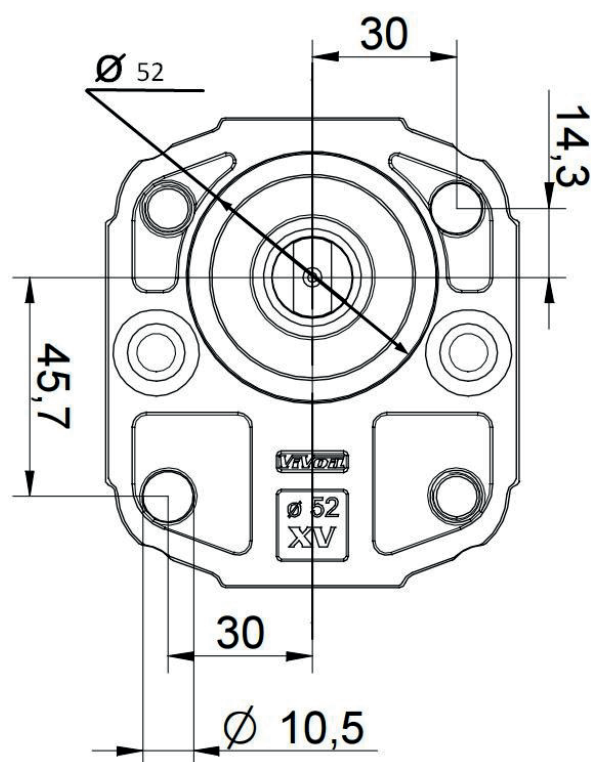
XV2 Ø52 BH POMPA (200.0256.XKP)
