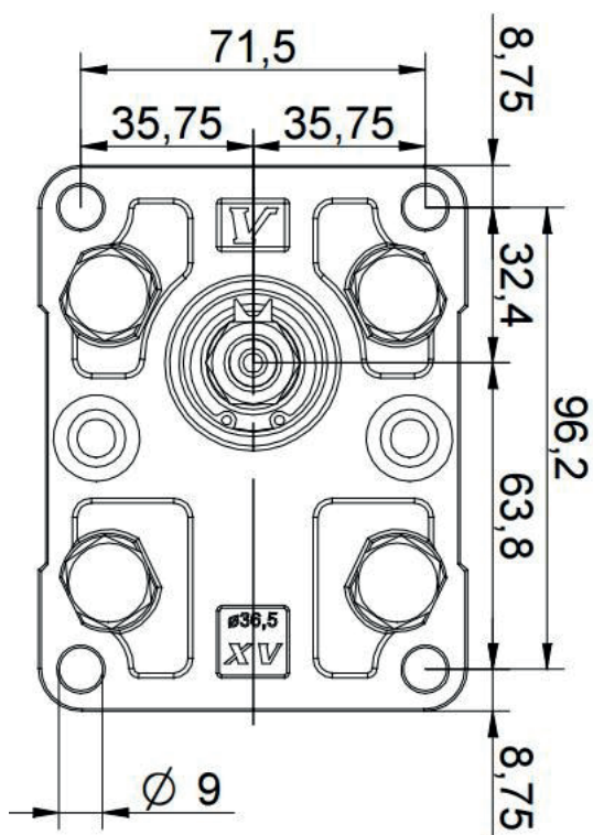
XV2 Ø36,5 (200.0241.XKP)
